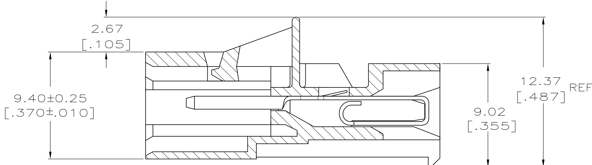
SECTION A-A
