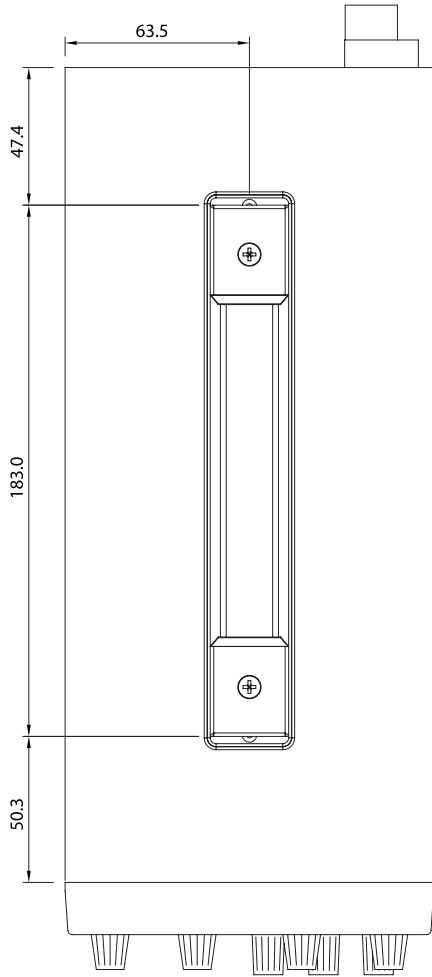
Dimensions : Millimetres
