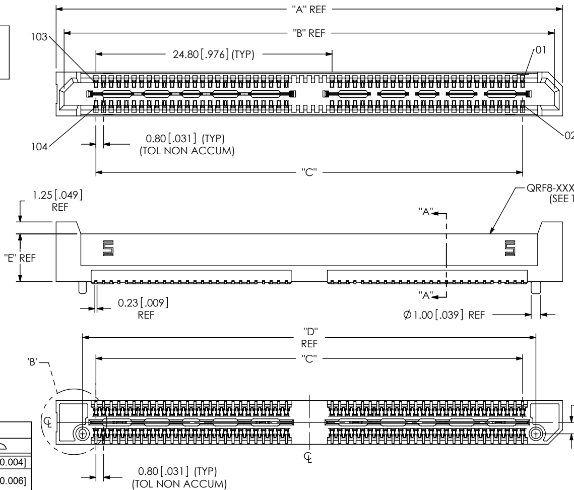
FIG 1 (QRF8-052-05.0-X-D-A SHOWN)
