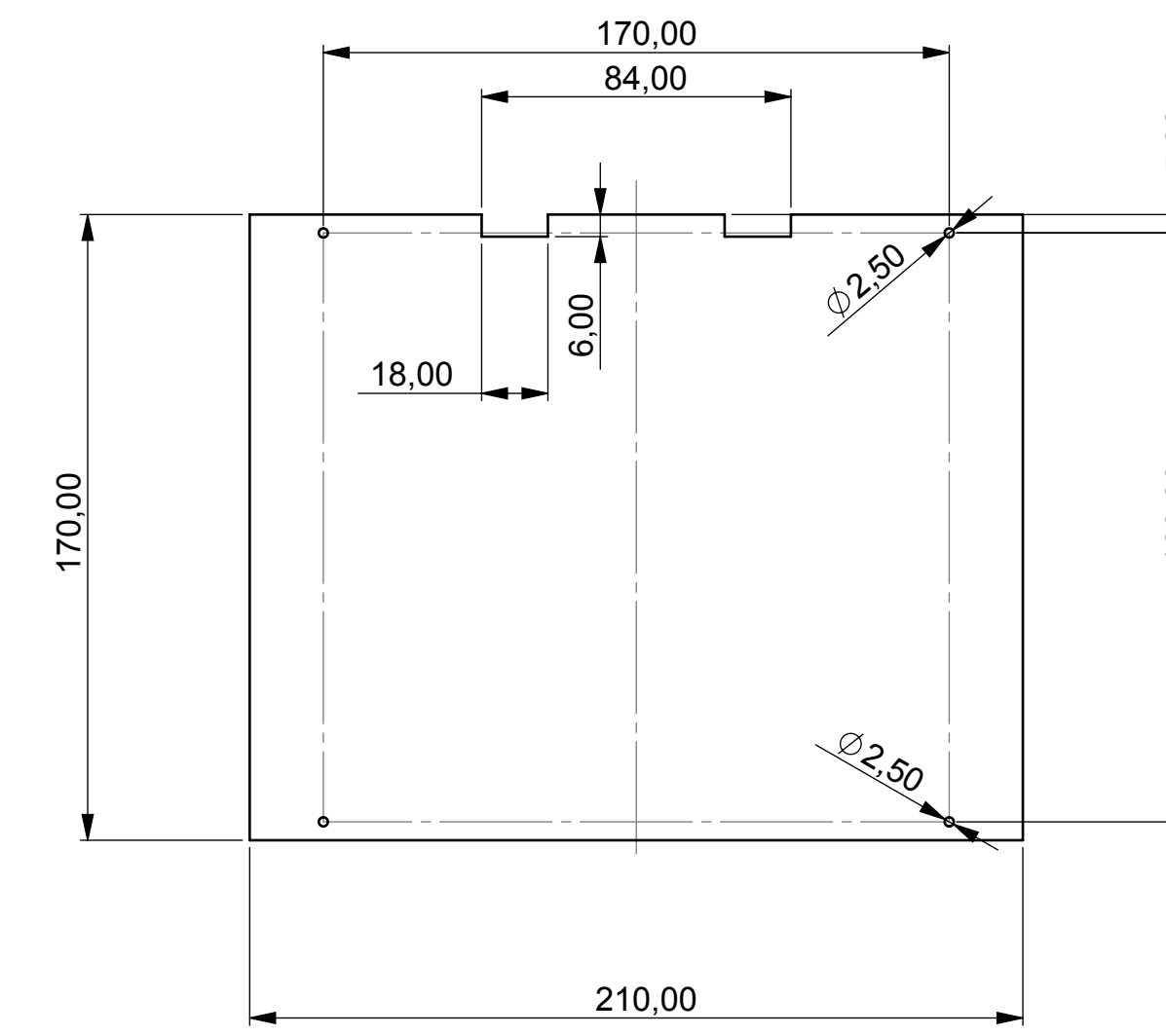
Platine Unterteil P C B Bottom Part
