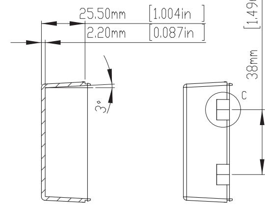
SECTION B-B SCALE 2 : 3
