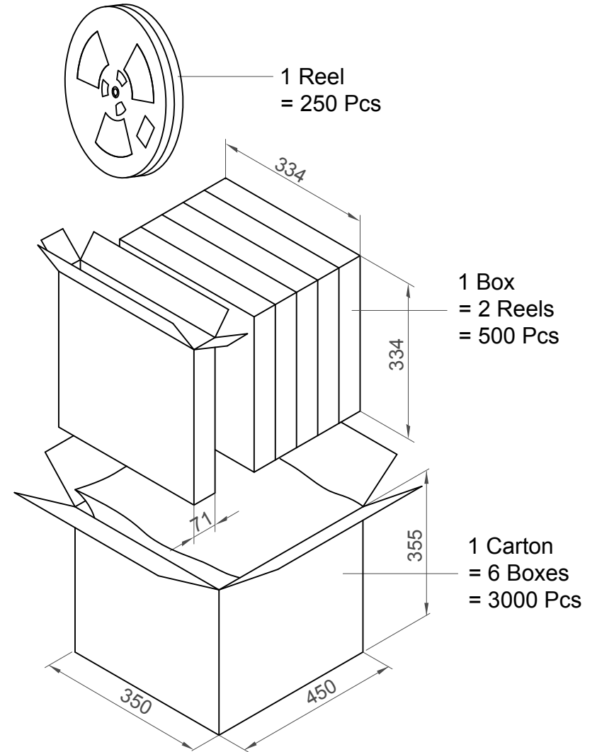
Reel 外觀尺寸圖 Fig 3.
