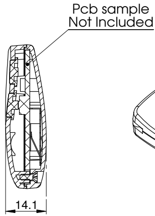
KESIT A-A
