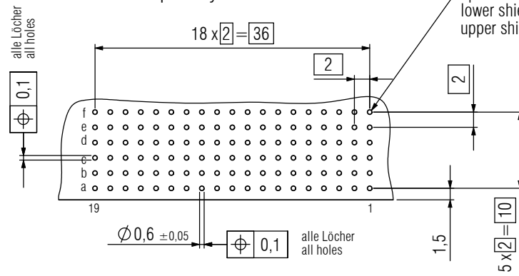
Leiterplatten-Lochbild pcb-layout
