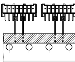
(8 極) (8 CKT.)
