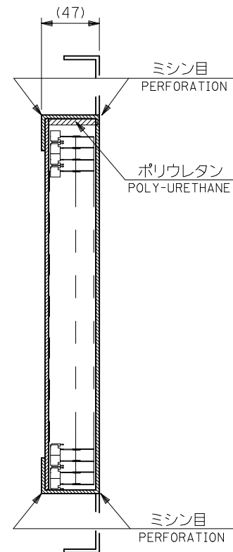
包装状態図 PACKAGING FORM
