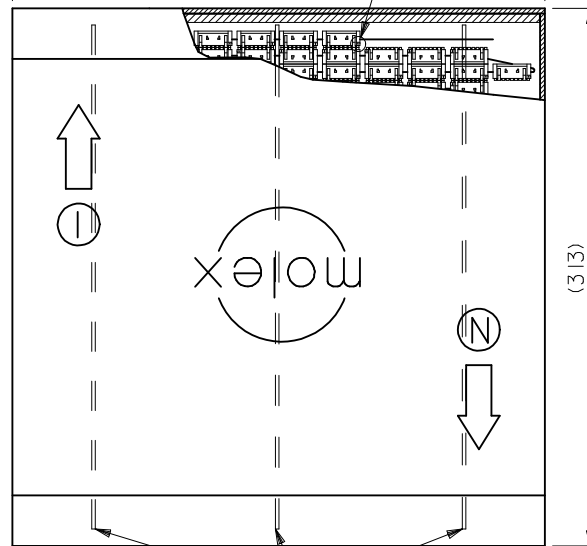
包装状態図 PACKAGING FORM
