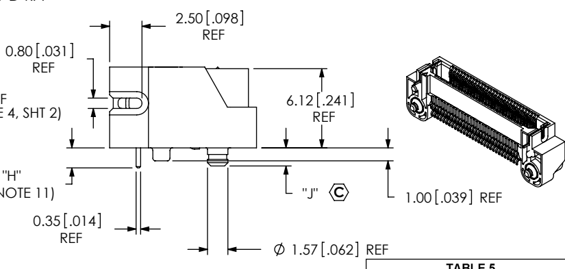
FIG 1 ERF8-030-01-X-D-RA SHOWN
