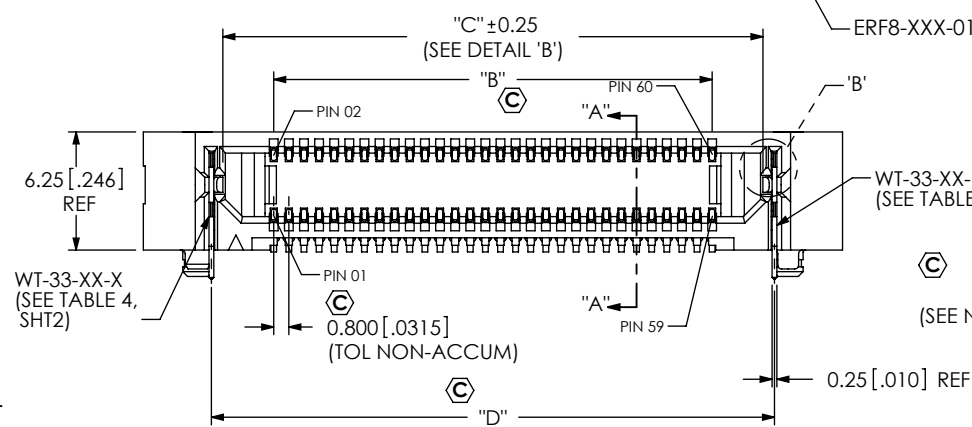
FIG 1 ERF8-030-01-X-D-RA SHOWN
