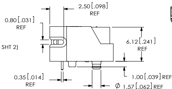
FIG 1 ERF8-030-01-X-D-RA SHOWN
