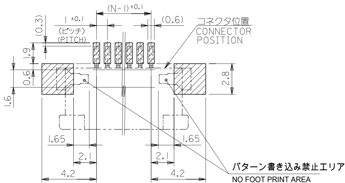
推奨基板レイアウト RECOMMENDED P.C. BOARD PATTERN DIMENSION.(REF.) (マウント面) (MOUNT SIDE)
