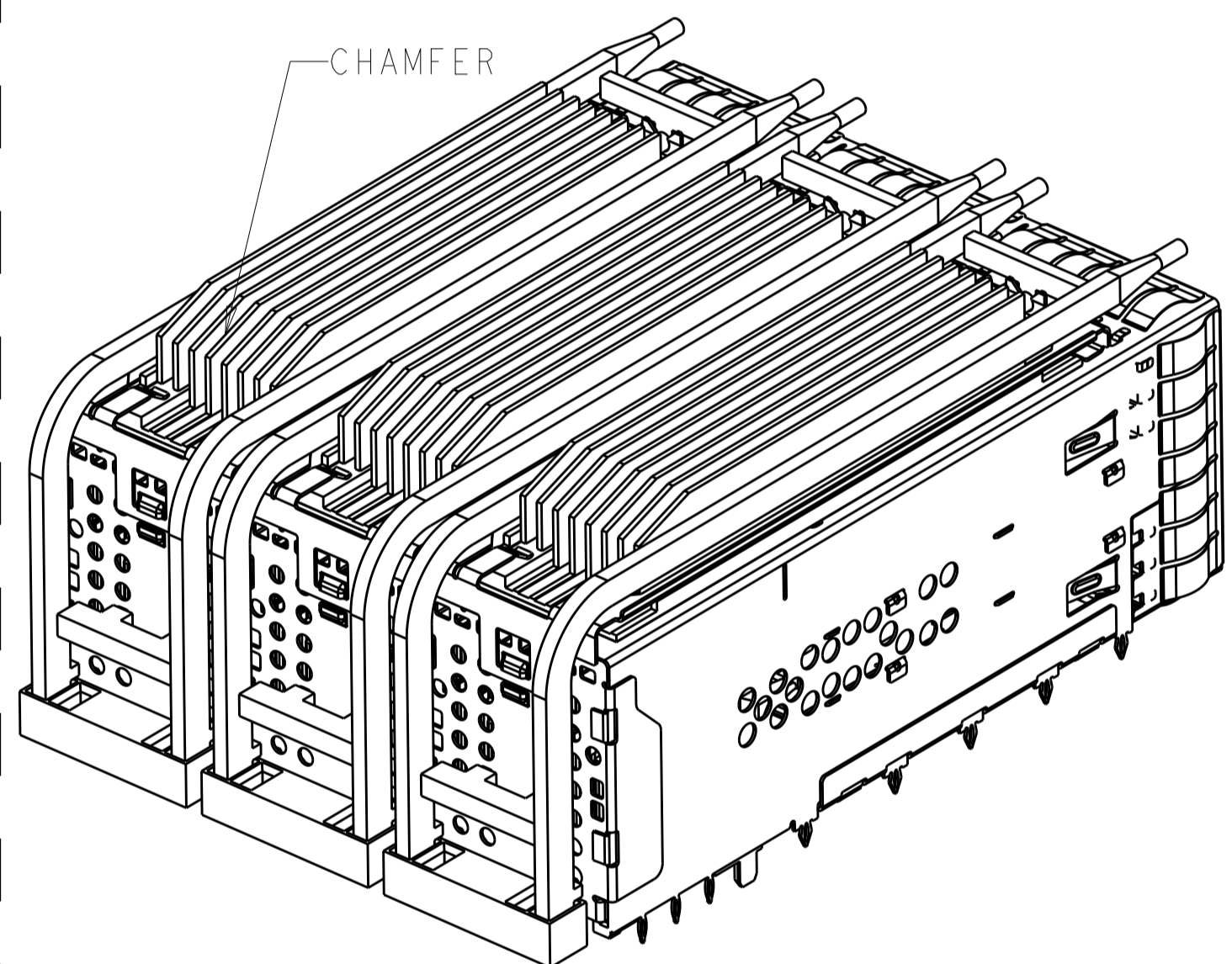
1-2299924-6 SCALE 2:1
