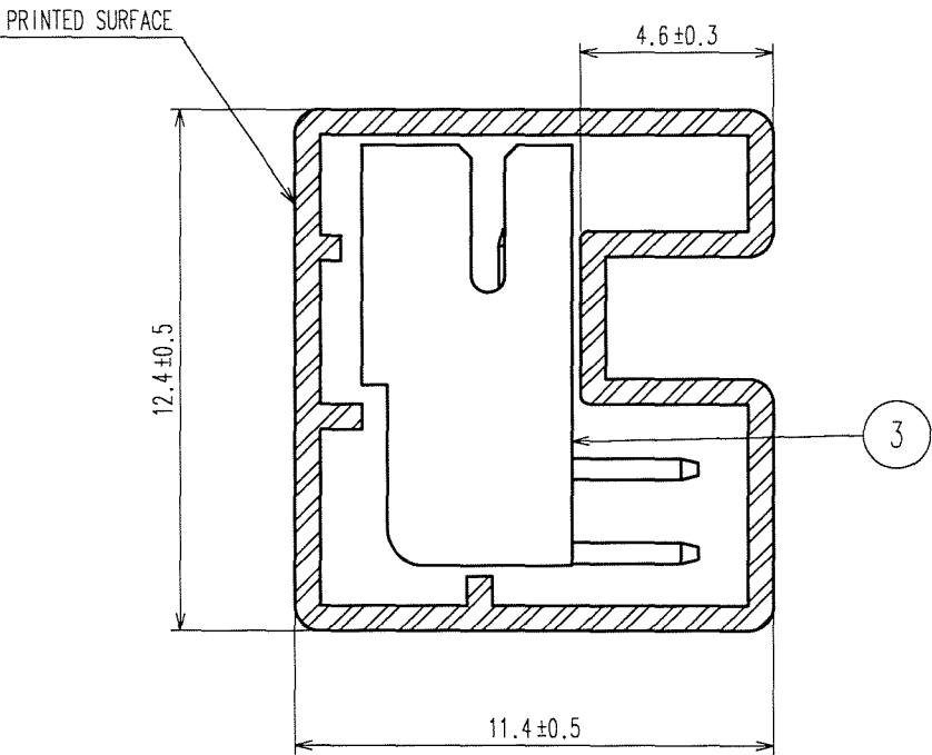
A-A (5:1)
