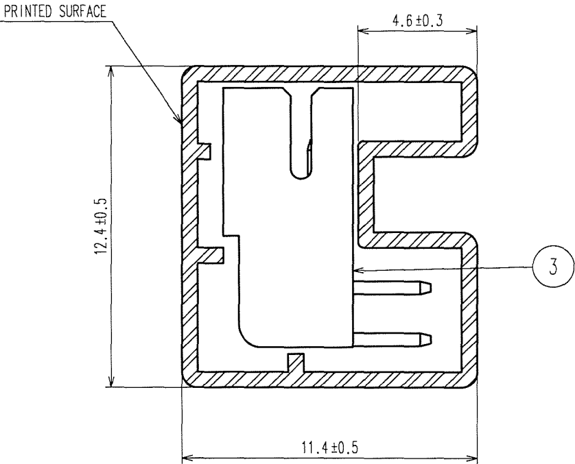
A-A (5:1)
