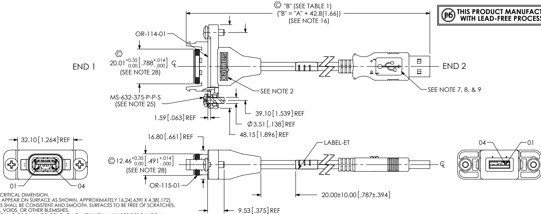
FIG 1 RPCU-X-XX.XX-AMS-AM SHOWN
