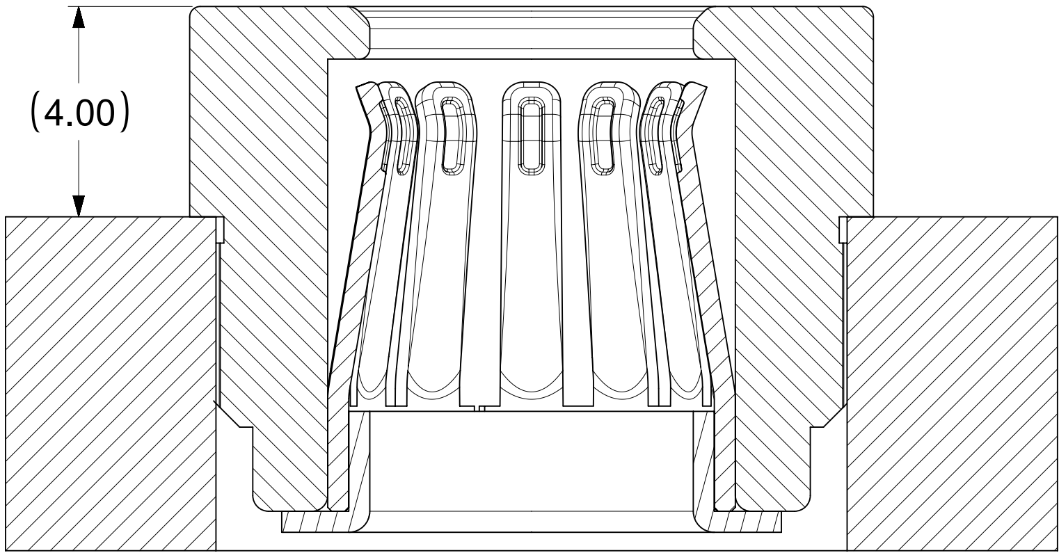
SECTION A-A
