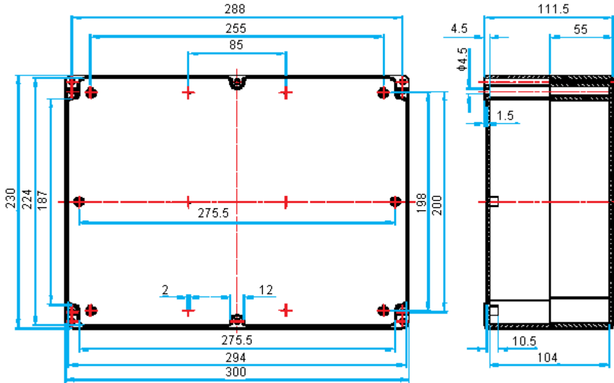
Dimensions : Millimetres
