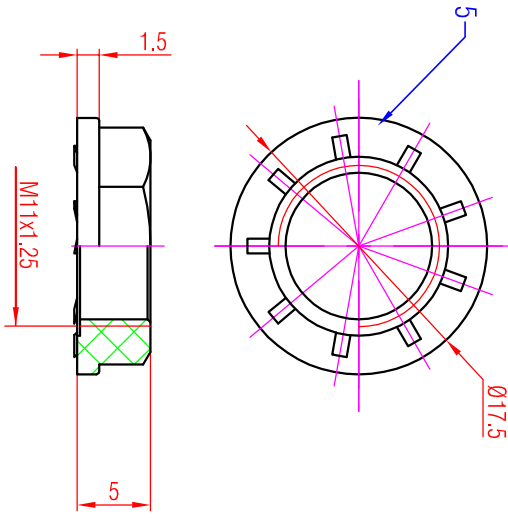
Nut
