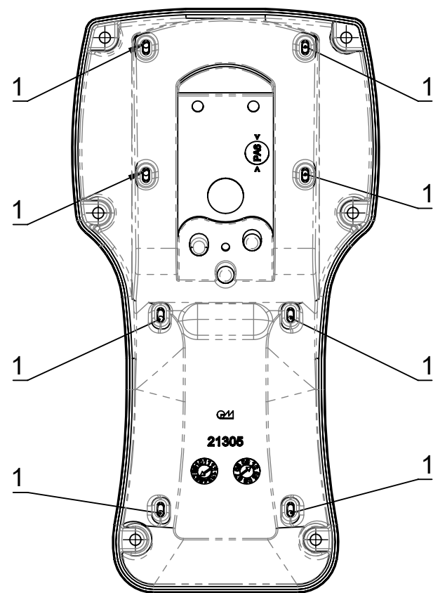
Unterschale/ enclosure bottom
