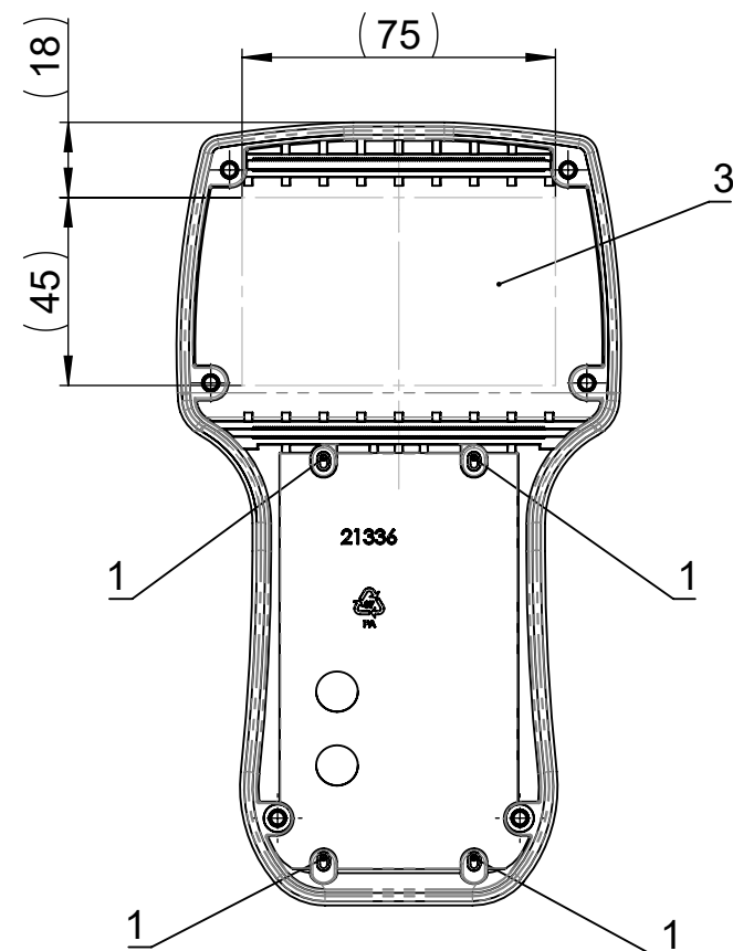
Oberschale/ enclosure top
