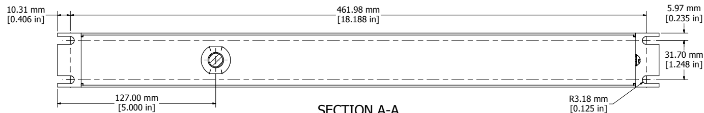
SECTION A-A
