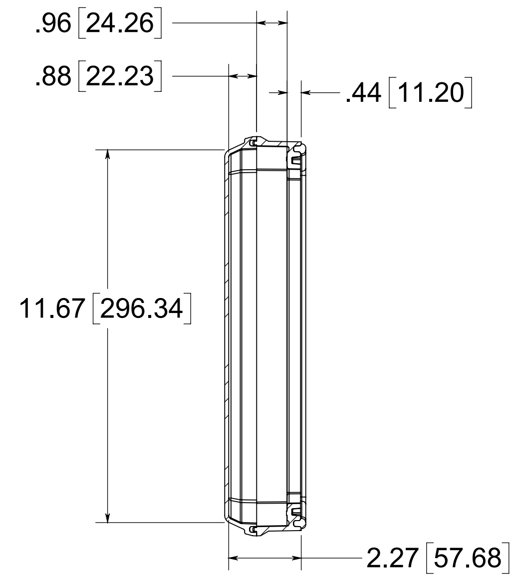
SECTION A-A
