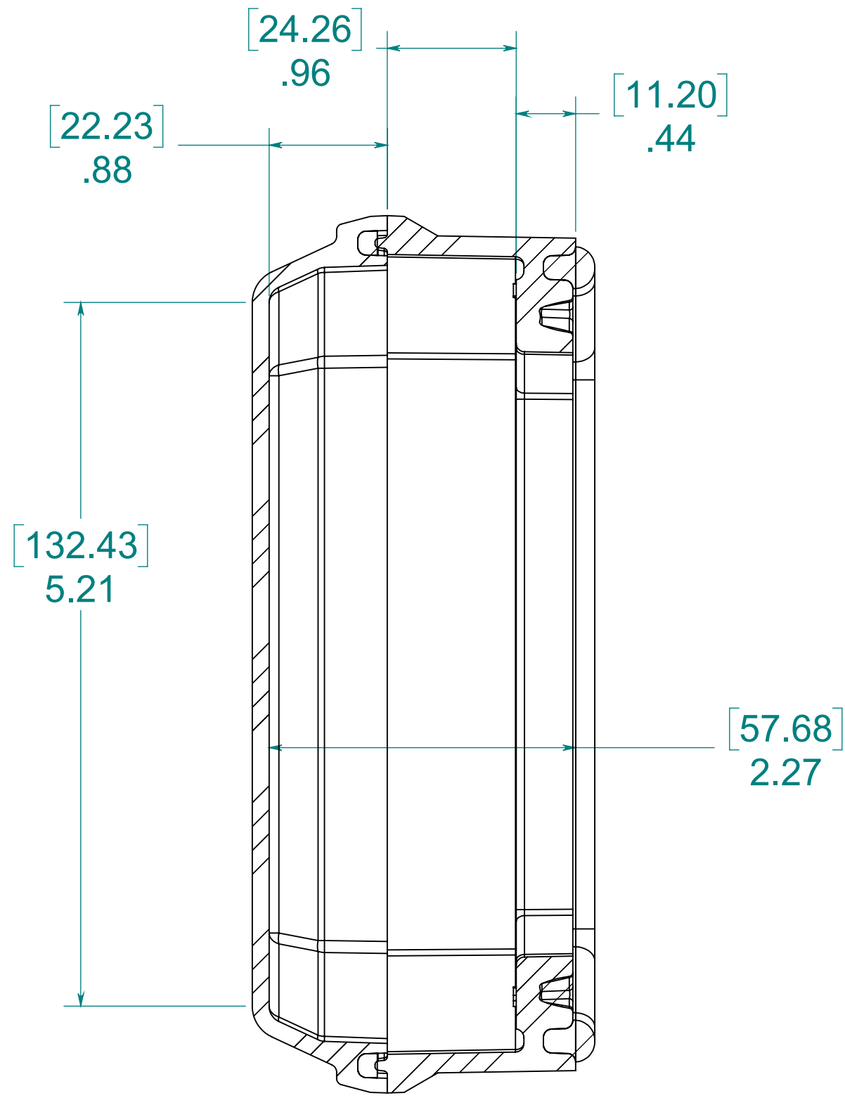
SECTION A-A
