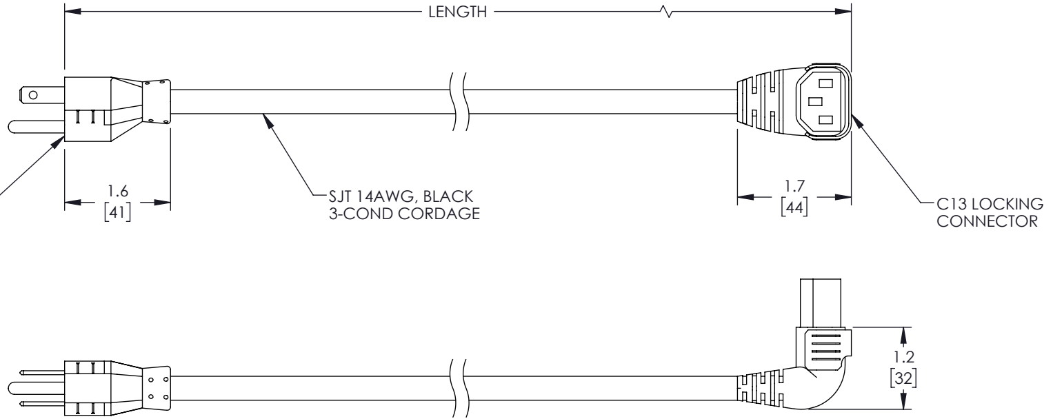
NEMA 5-15P PLUG
