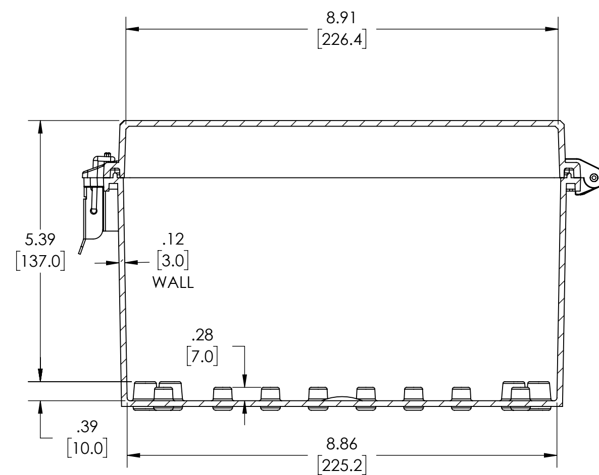
SECTION A-A
