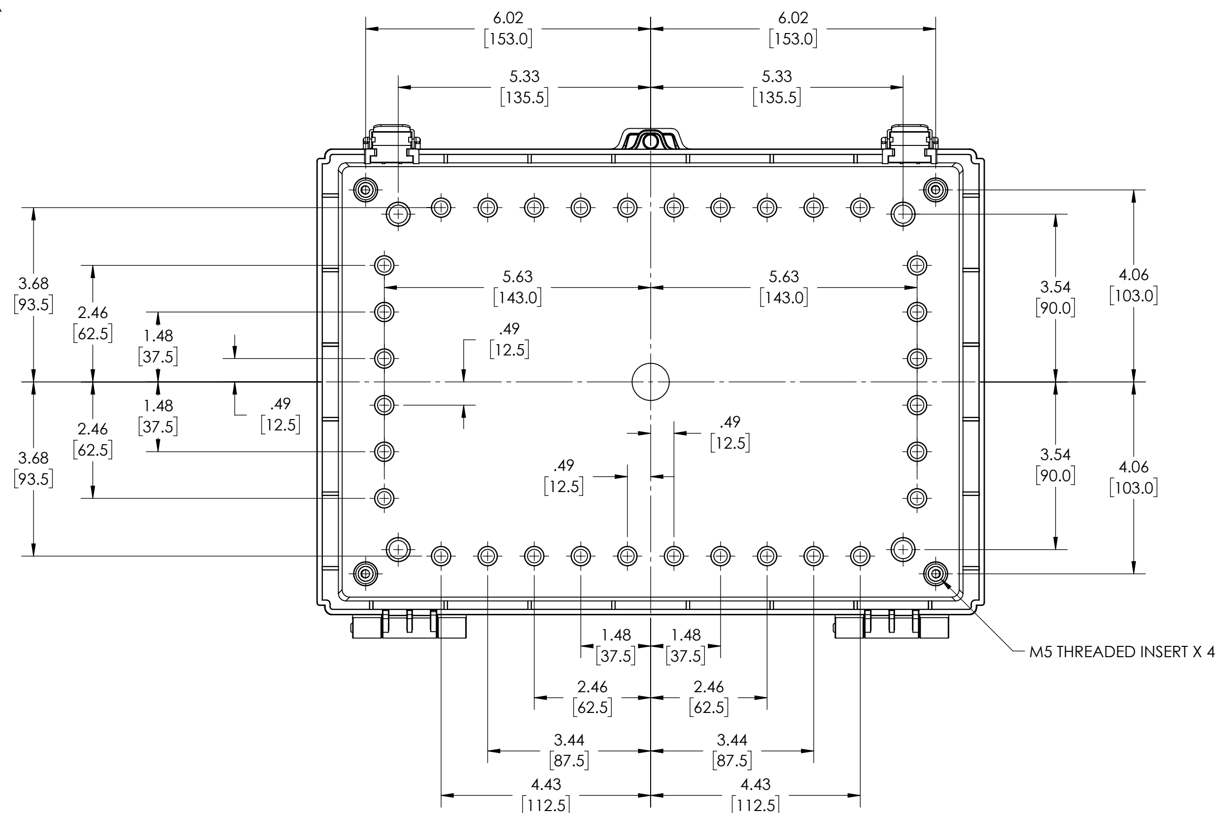
SECTION A-A
