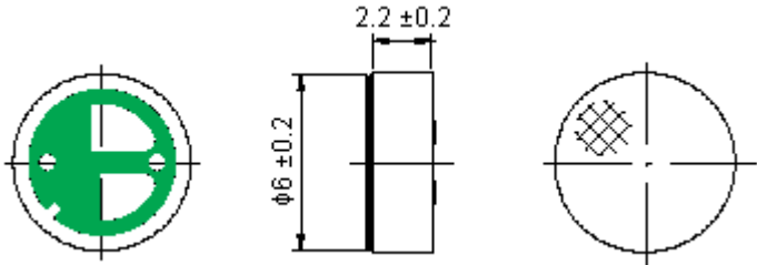
Dimensions : Millimetres
