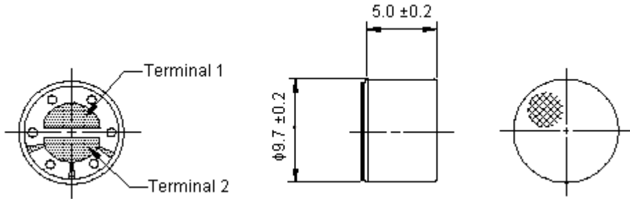
Dimensions : Millimetres
