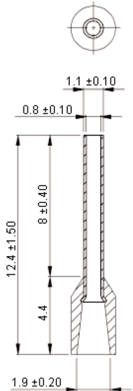
Dimensions : Millimetres
