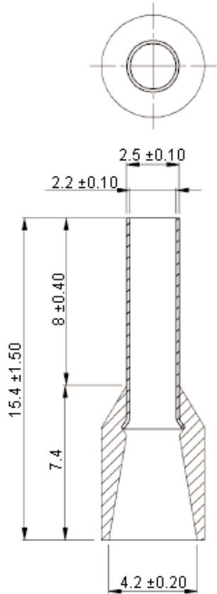
Dimensions : Millimetres
