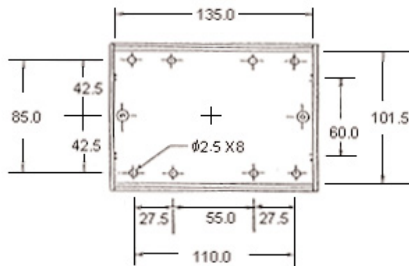
Dimensions : Millimetres
