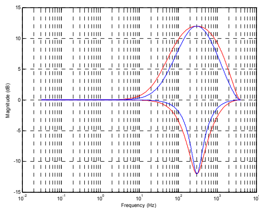
Figure 60 EQ Band 4 – EQ3BW=0, EQ3BW=1
