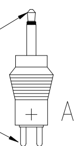
Klinkenstecker/ jackplug ø2,5x12mm
