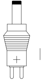
Hohlstecker/ hollowplug ø2,5xø5,5x12mm
