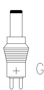
Klinkenstecker/ jackplug ø3,5x15mm
