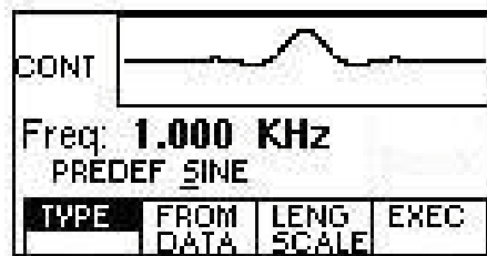
Predefine Menu
