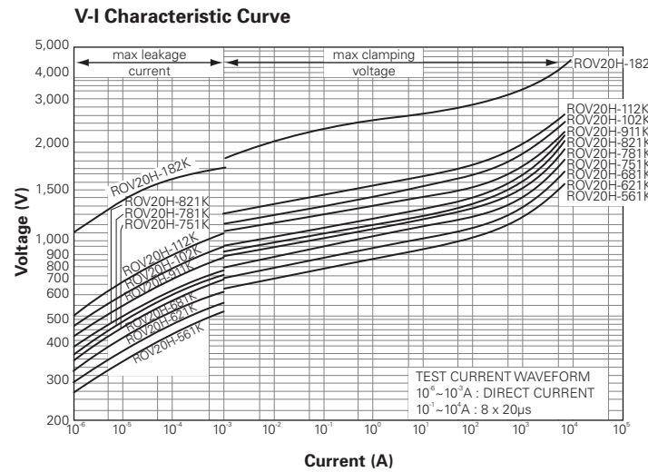
Figure V28 - ROV20H561K-ROV20H182K
