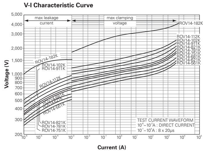
Figure V12 - ROV14-561K-ROV14-182K
