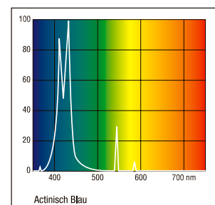
Coralstar
