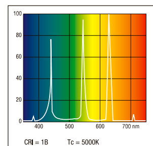
Daylightstar
