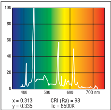
Activa® 172
