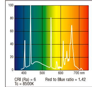
Gro-Lux
