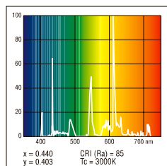
Warmwhite Deluxe 830
