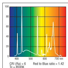
Gro-Lux®
