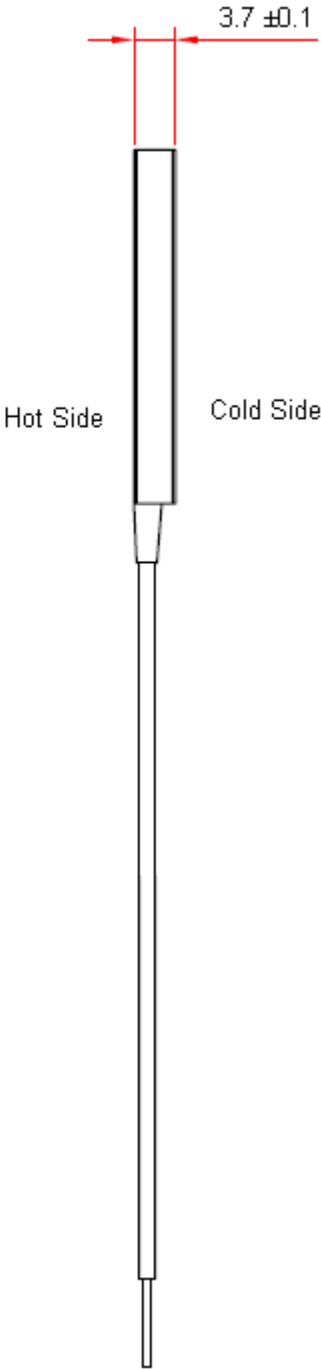
Dimensions : Millimetres
