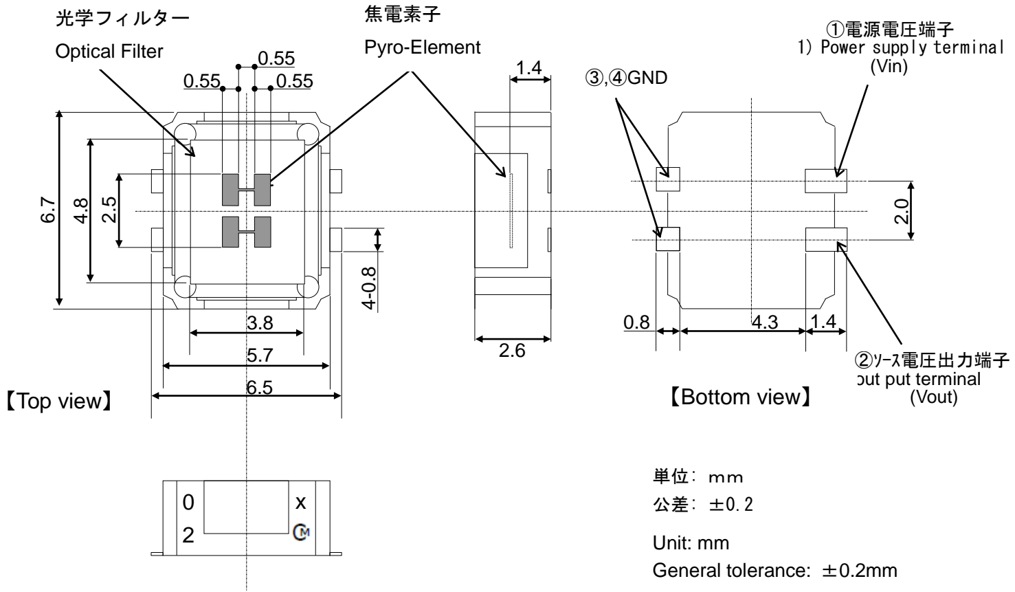
図1 形状及び寸法 Figure 1. Outline Dimensions
