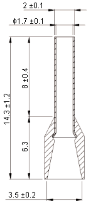
Dimensions : Millimetres
