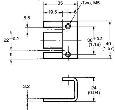
Y92E-C20
