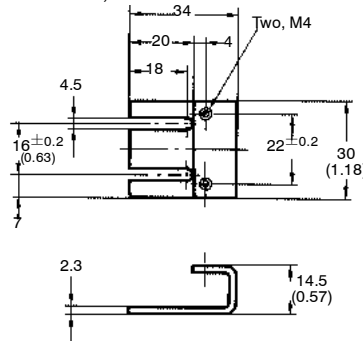
Y92E-C10
