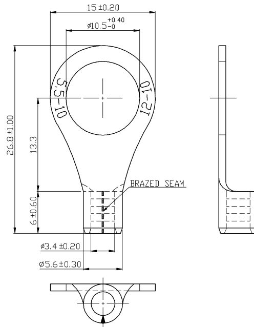
Dimensions : Millimeters
