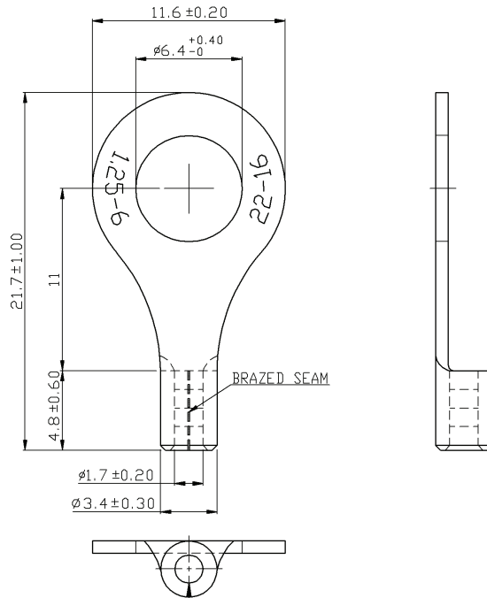
Dimensions : Millimeters
