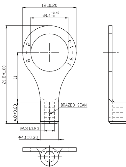
Dimensions : Millimeters
