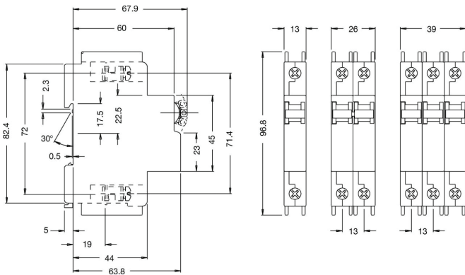
Dimensions : Millimeters
