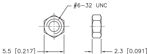
Nut
