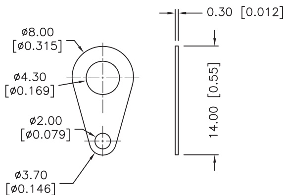
Solder Lug
