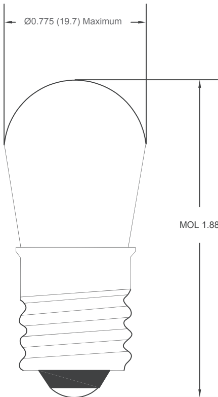
Dimensions : Inches
