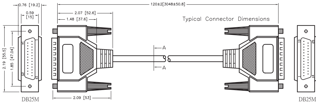
Dimensions : Millimeters (Inches)
