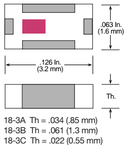
Case 18-3 (EIA 1206 / 3216)
