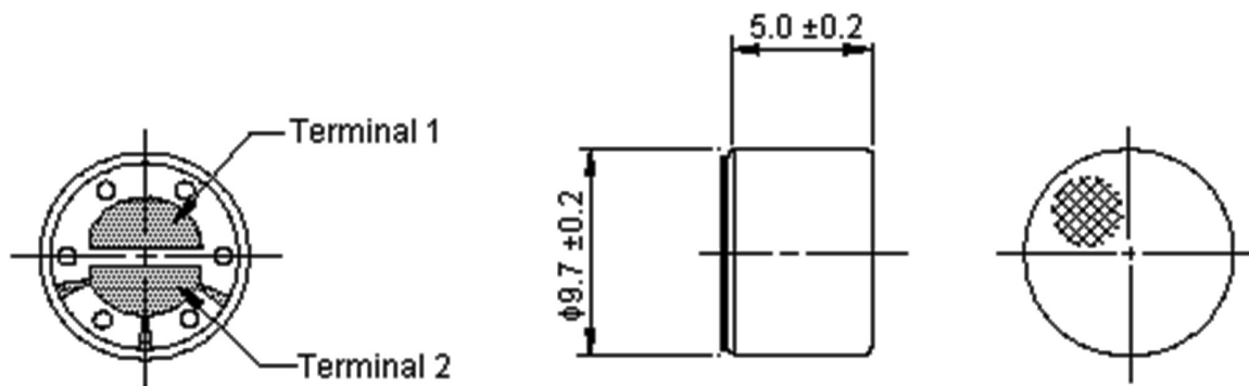
Dimensions : Millimetres
