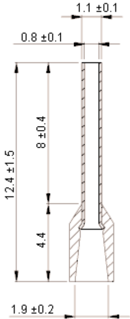
Dimensions : Millimetres
